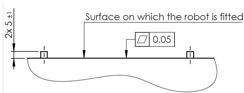
1.2: Montážní deska pro základnu robota
